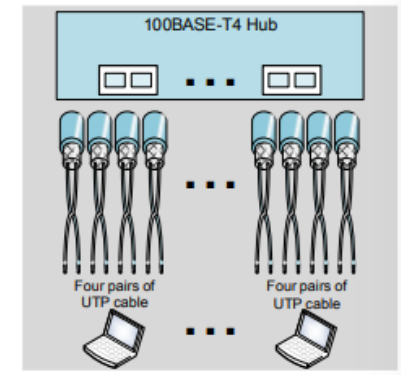
C. 100BASE-T4
