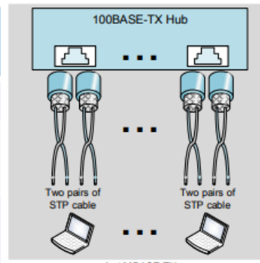
A. 100BASE-TX
