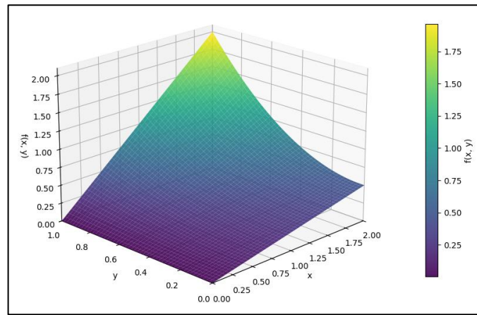
<그림 19> 예제 3.19 f(x, y) 의 결합확률밀도함수도
