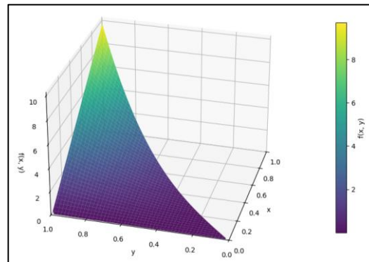
<그림 15> 예제 3.18 f(x, y) 의 결합확률밀도함수도
