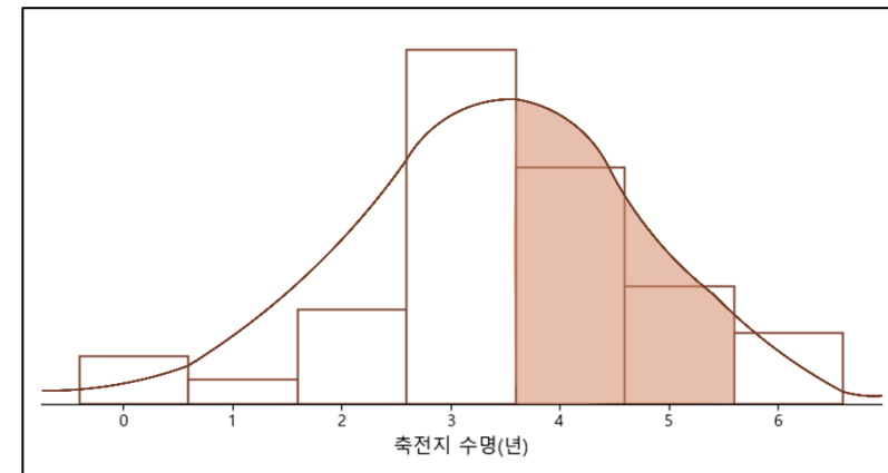
▲ 확률밀도함수의 추정
