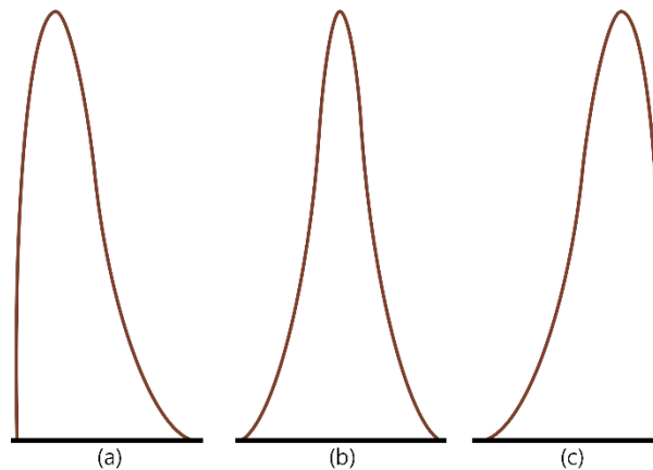
<그림 8> 자료의 기움(왜도) 그래프 모형
