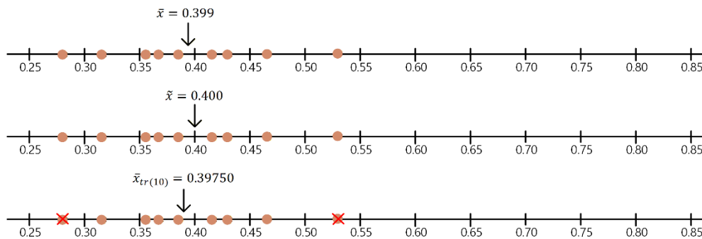
▲ 무질소 표본에 대한 위치측도
