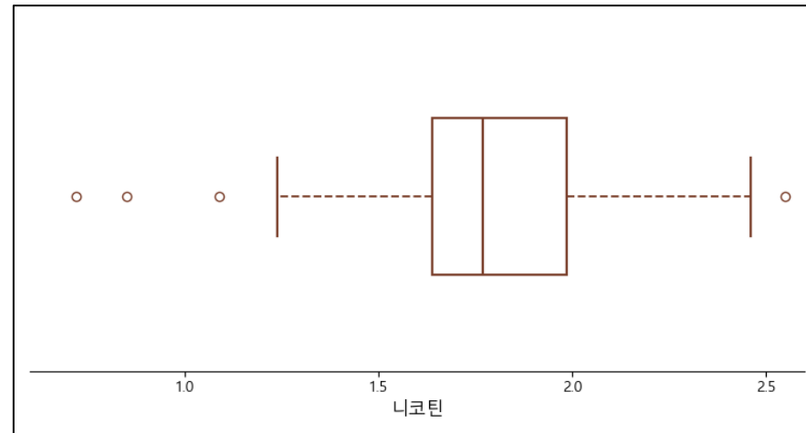
<그림 9> 니코틴 자료에 대한 상자-수염 그림
