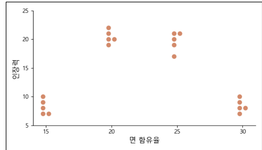
<그림 3> 면 함유율과 인장력의 산점도 그래프
