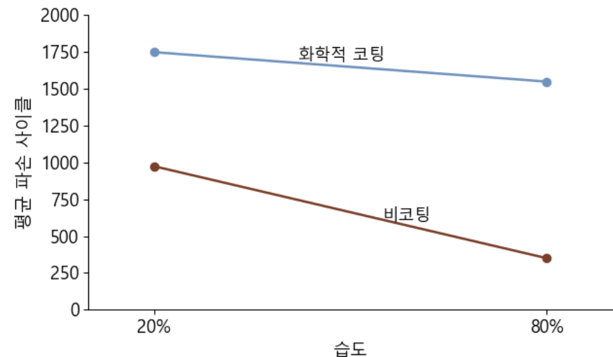
<그림 2> 예제 1.3의 부식 결과 그래프
