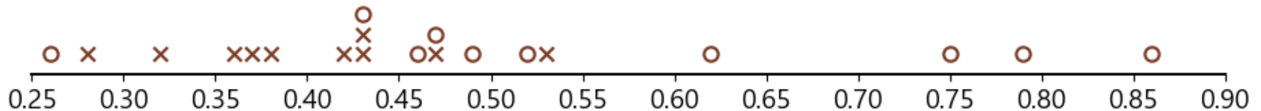
<그림 1> 줄기 무게의 점도표
