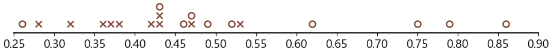
<그림 1> 줄기 무게의 점도표
