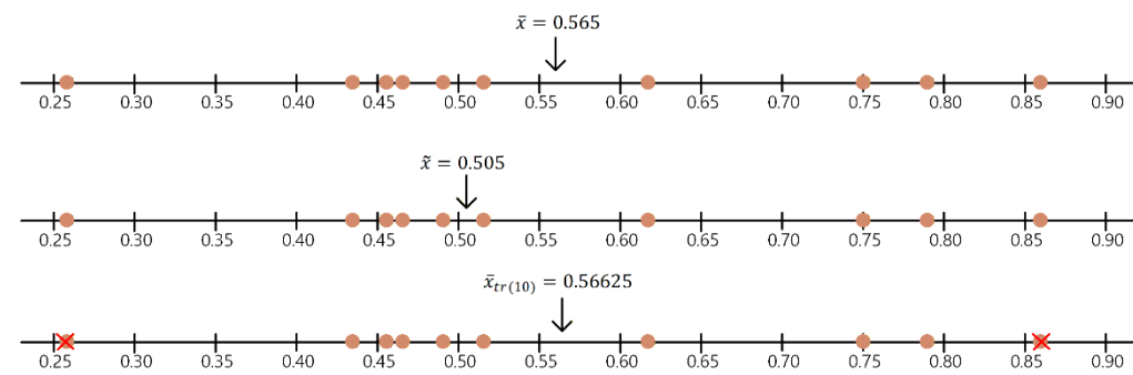
▲ 질소 표본에 대한 위치측도
